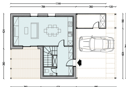
TLORIS PRITLIČJA 37,45 m 2
