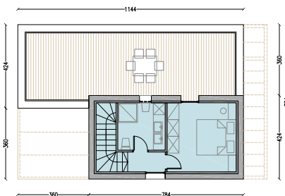
TLORIS NADSTROPJA 24,85 m 2
